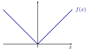
Example 5.2 (v): f(x) = |x|
