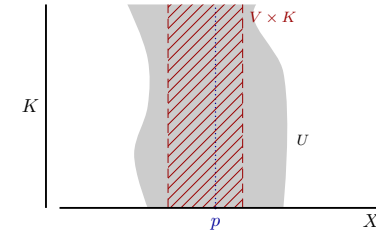
FIGURE 8.4: Tube lemma (Lemma 8.31).
